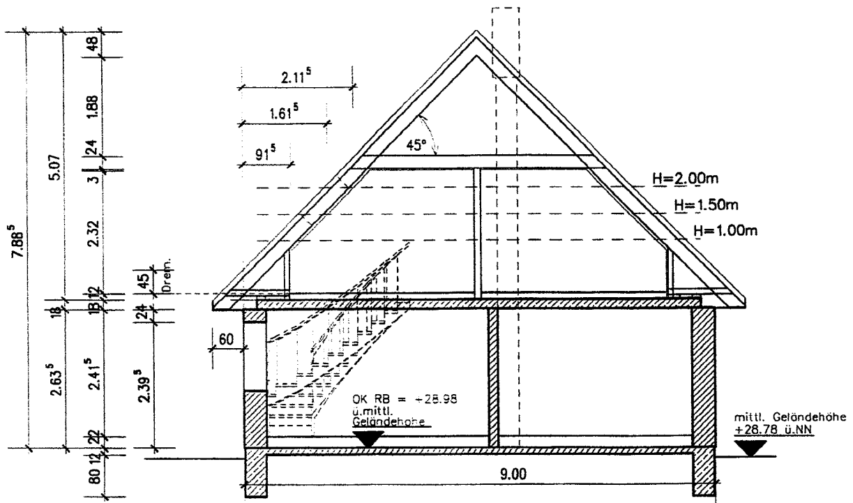
Schnitt
